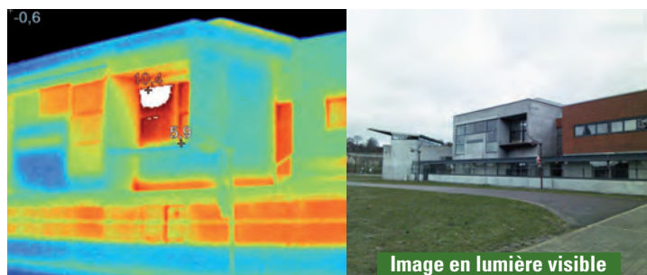
04/12/2020 08:46:48. Des ponts thermiques sont visibles entre chaque élément de maçonnerie.
