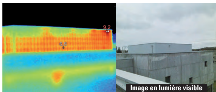
04/12/2020 09:32:36 : Des déperditions thermiques sont visibles sur le bardage
